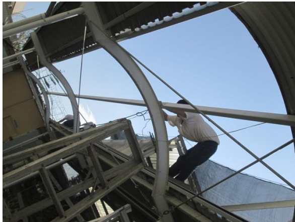
吊掛鐵皮屋頂
